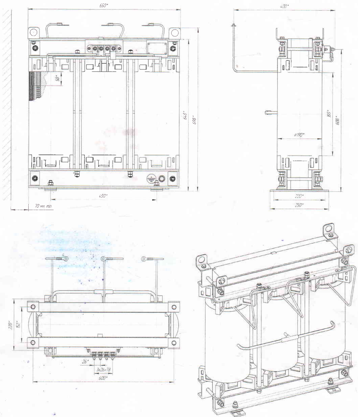
Рисунок 1 - Общий вид, габаритные, установочные и присоединительные размеры трансформатора типа ТСКК-25/10 – У3. Масса трансформатора 270 кг.
